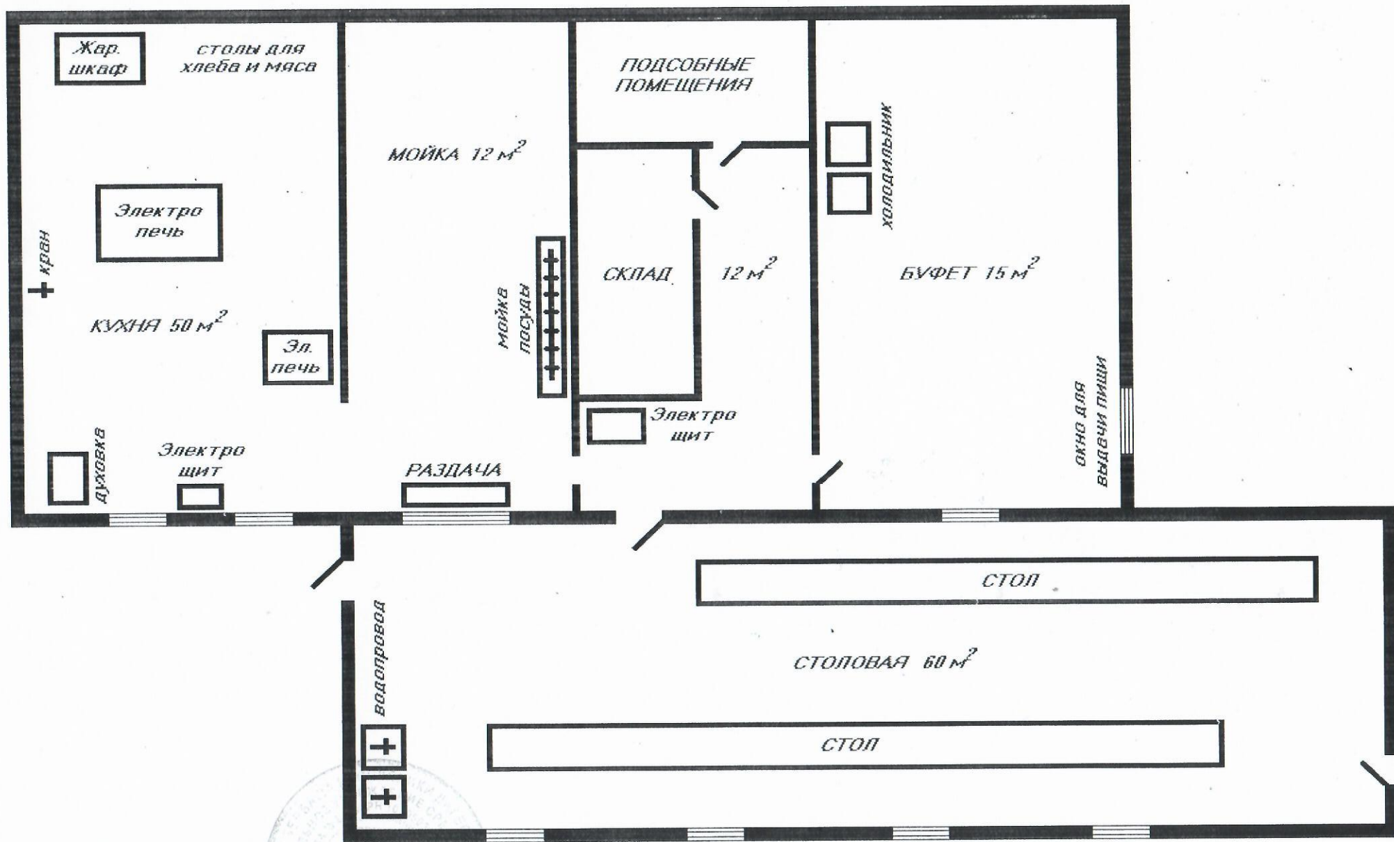
ПЛАН-СХЕМА ПИЩЕБЛОКА СОШ №8 В. З.
